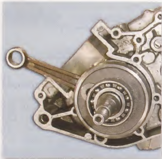
Vistas del carter de motor dos tiempos
